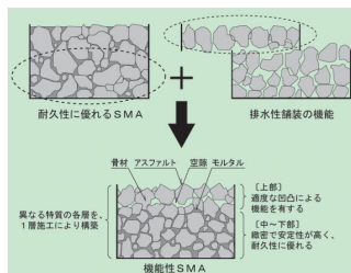
機能性SMAの概要
