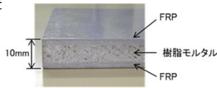
断面構成
