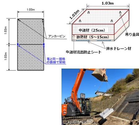
施工の様子
