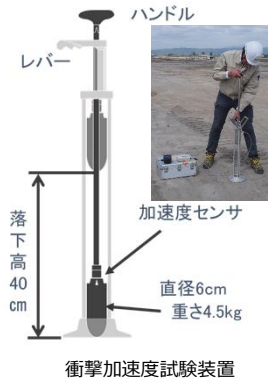
衝撃加速度試験装置
