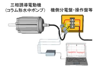
電流情報診断による計測方法
