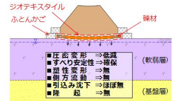
グラベル基礎補強工法による対策効果
