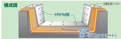
断面構成図
