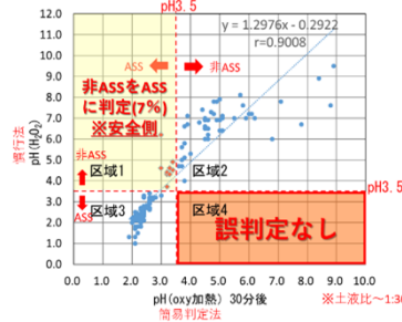
従来法（慣行法）と簡易判定法との関係
