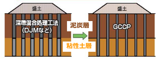
工法概略図
