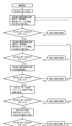
泡流出時の対処フロー
