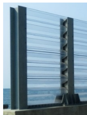
道路側から見た柵の形状
