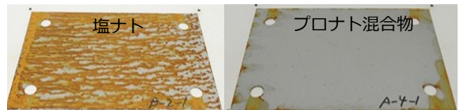
試験片の金属腐食状況（北陸東海自動車道での比較試験）
