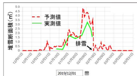
堆雪断面面積の推計グラフ
