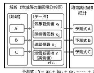
堆雪断面面積の解析手法
