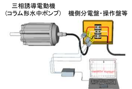
電流情報診断による計測方法
