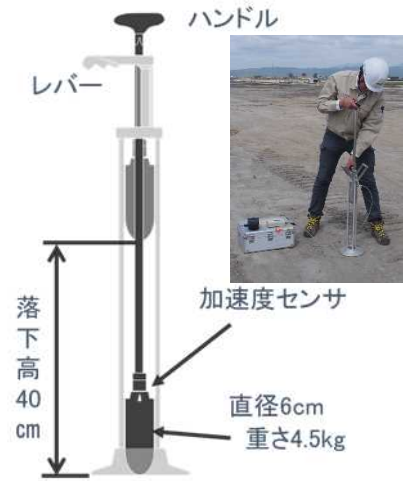
衝撃加速度試験装置
