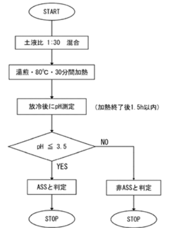
簡易判定法の判定フロー図
