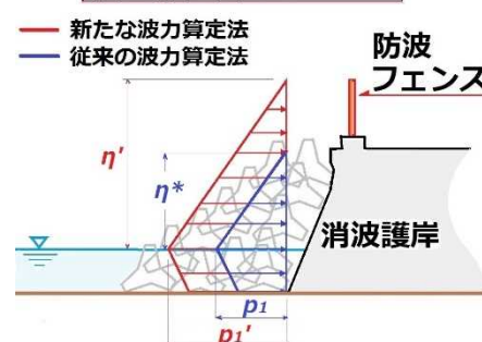
防波フェンスに作用する波力のイメージ図
