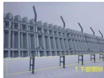
設置状況（石狩吹雪実験場）
