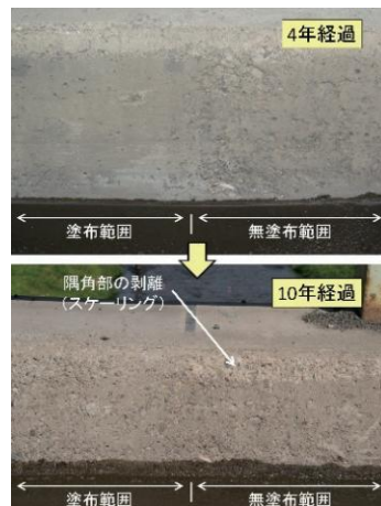
シランの効果
