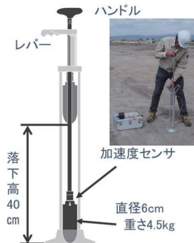
衝撃加速度試験装置
