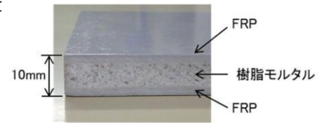
断面構成
