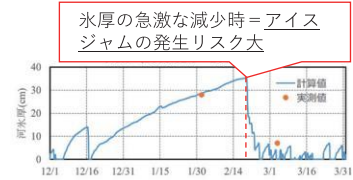
アイスジャムの予測例
