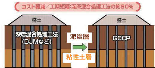
工法概略図
