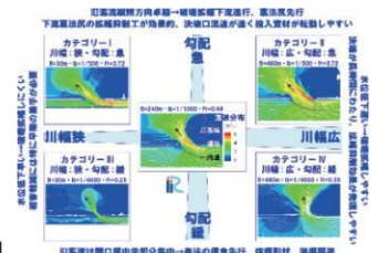
河道形状に応じた 堤防決壊現象の分類図
