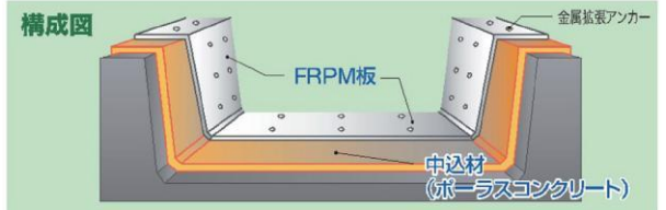
断面構成図
