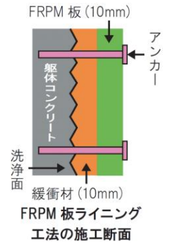
FRPM板ライニング工法の施工断面
