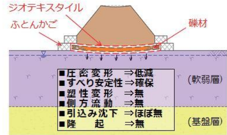
グラベル基礎補強法による対策効果
