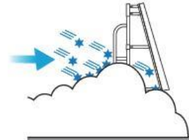
下部間隙閉塞時、柵風上に雪粒子を捕捉
