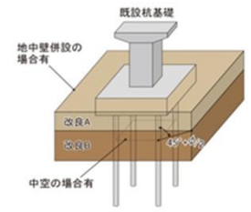
工法概略図
