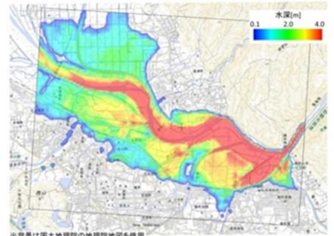
氾濫の再現計算 （2013年9月 亀岡市）
