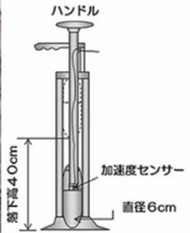
衝撃加速度試験装置
