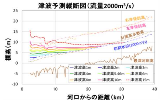
津波予測縦断面図（流量2000m³/s）
