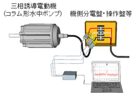
電流情報診断による計測方法
