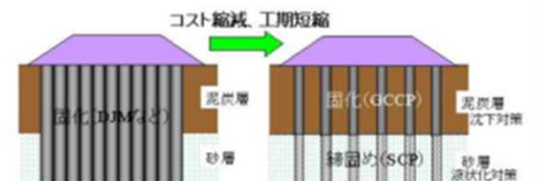
工法概略図
