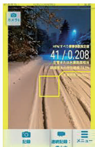
AI画像認識技術を用いた路面のすべり摩擦係数の推定システムの開発
