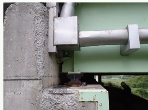
橋上に生じたスケーリング
