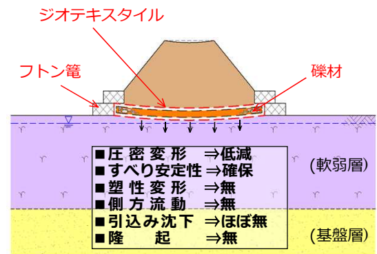
グラベル基礎補強工法による対策効果
