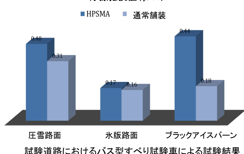
摩擦抵抗値 (μ 30)
