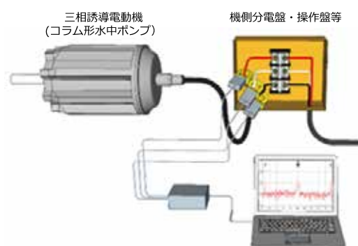
電流情報診断による計測方法
