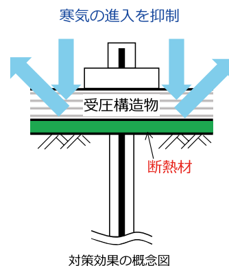
対策効果の概念図
