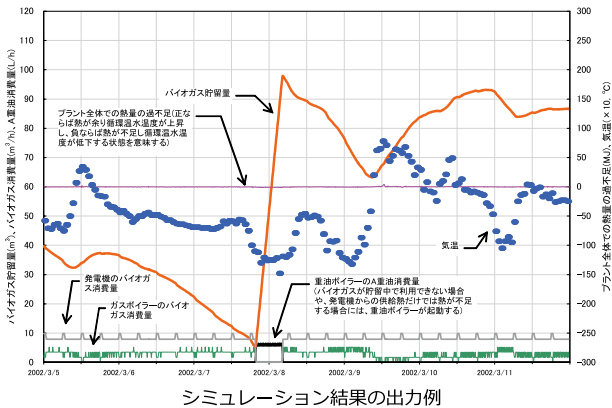
シミュレーション結果の出力例
