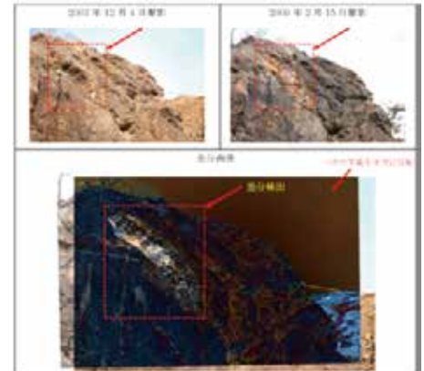
背景差分法の概要
