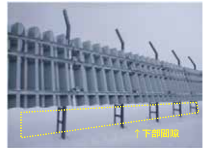
設置状況（石狩吹雪実験場）
