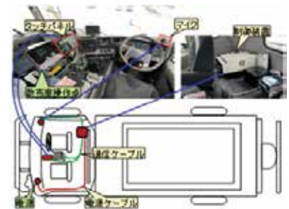
凍結防止剤散布車への搭載
