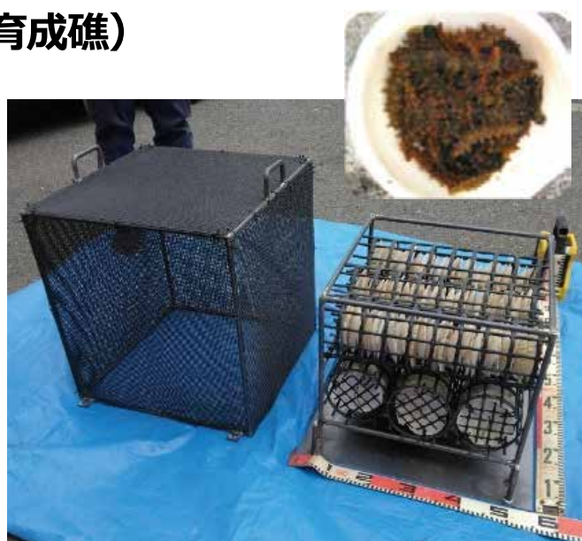
「ナマコのゆりかご」の外観
