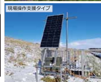
樋門監視システム設置状況
