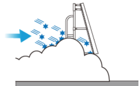
下部間隙閉塞時、柵風上に雪粒子を捕捉
