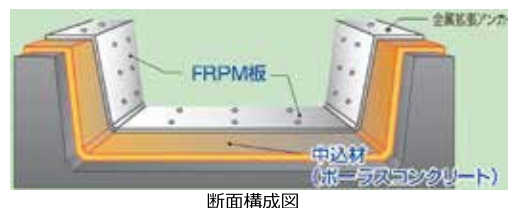
断面構成図
