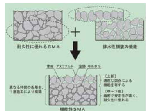
機能性SMAの概要
