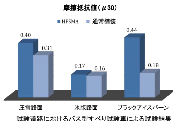
試験道路におけるバス型すべり試験車による試験結果
