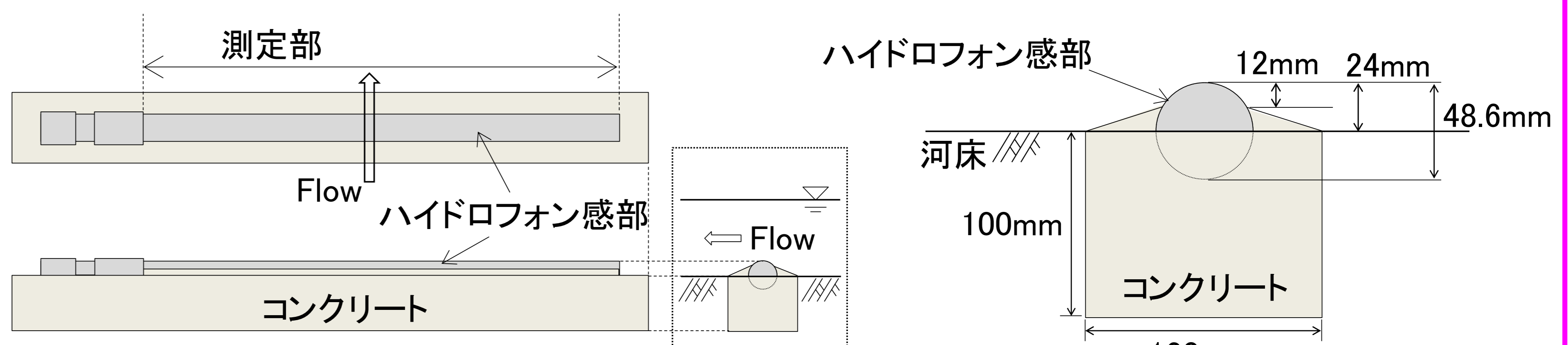
【掃流砂計の加工と現地設置状況】
