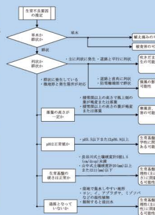
生育不良要因推定フロー図
