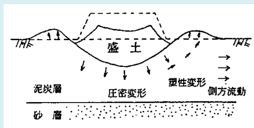
盛土による泥炭地盤の変形
