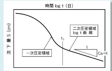
泥炭地盤の沈下挙動（概念図）
